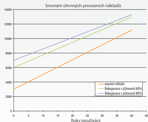
graf č. 2 – Provozní náklady a návratnost pro různé ventilační systémy Předpoklad: 1 kWh = 2,5 Kč + DPH
