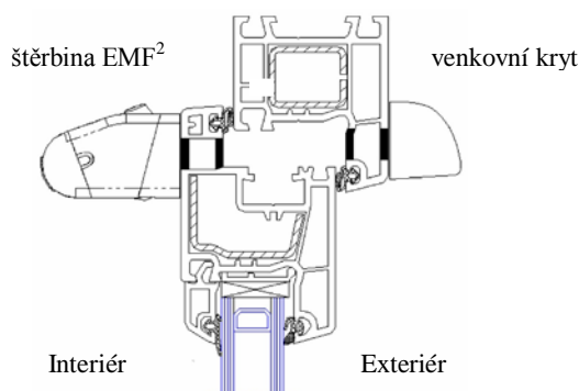
Řez plastového okna se štěrbinou
