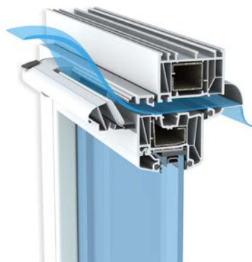
Instalace na plastovém okně
