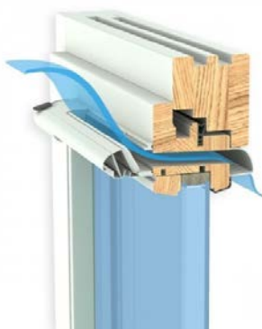
Instalace na dřevěném okně
